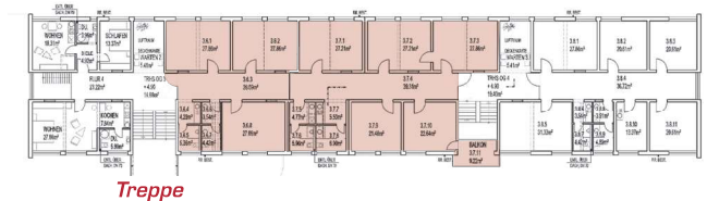
Haus 4, Obergeschoss
