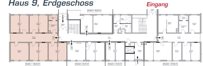
Haus 9, Erdgeschoss
